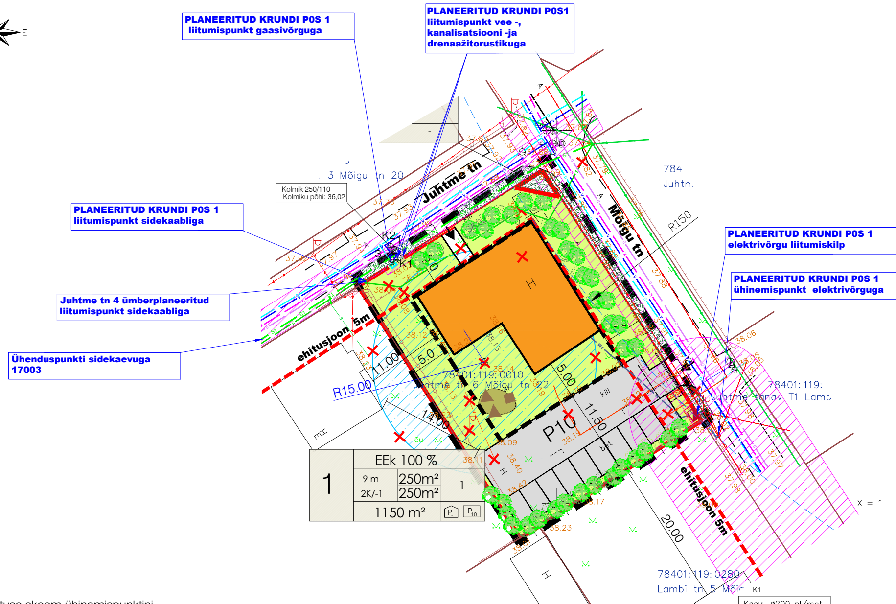
Sidevarustuse skeem ühinemispunktini
